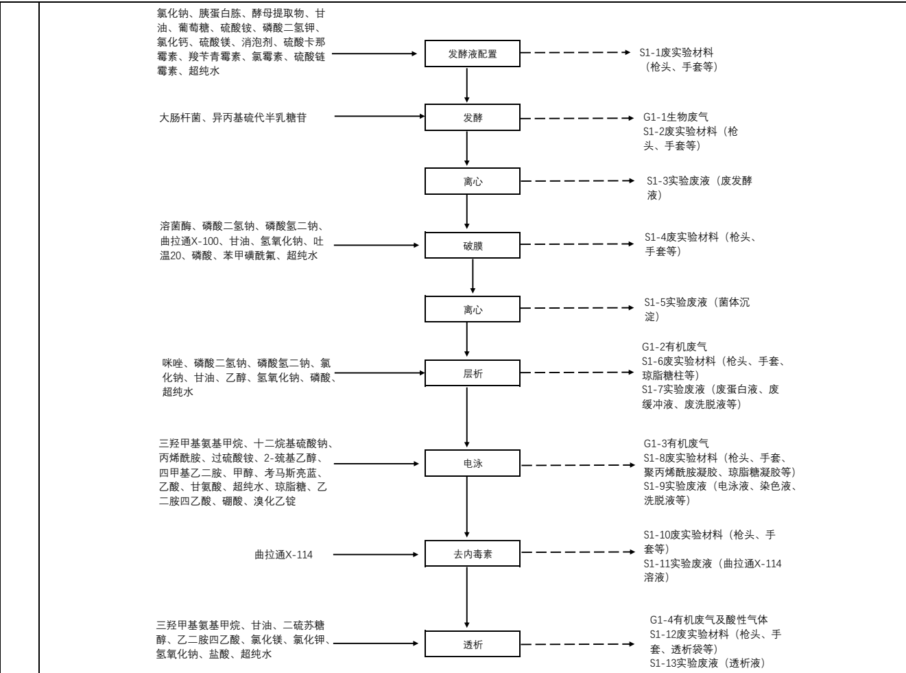
图 2-2 酶制品工艺流程图及产污环节
